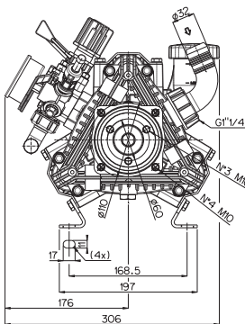
MI1 Flange
