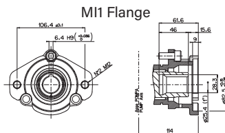
MI1 Flange
