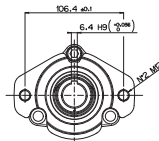
MI1 Flange
