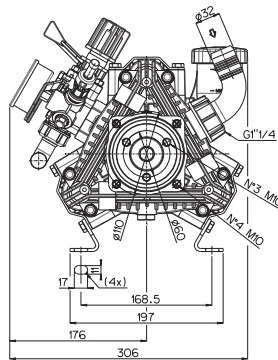
MI1 Flange
